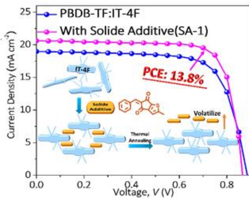
图：可挥发固体添加剂的工作机制示意图以及所优化的器件性能
