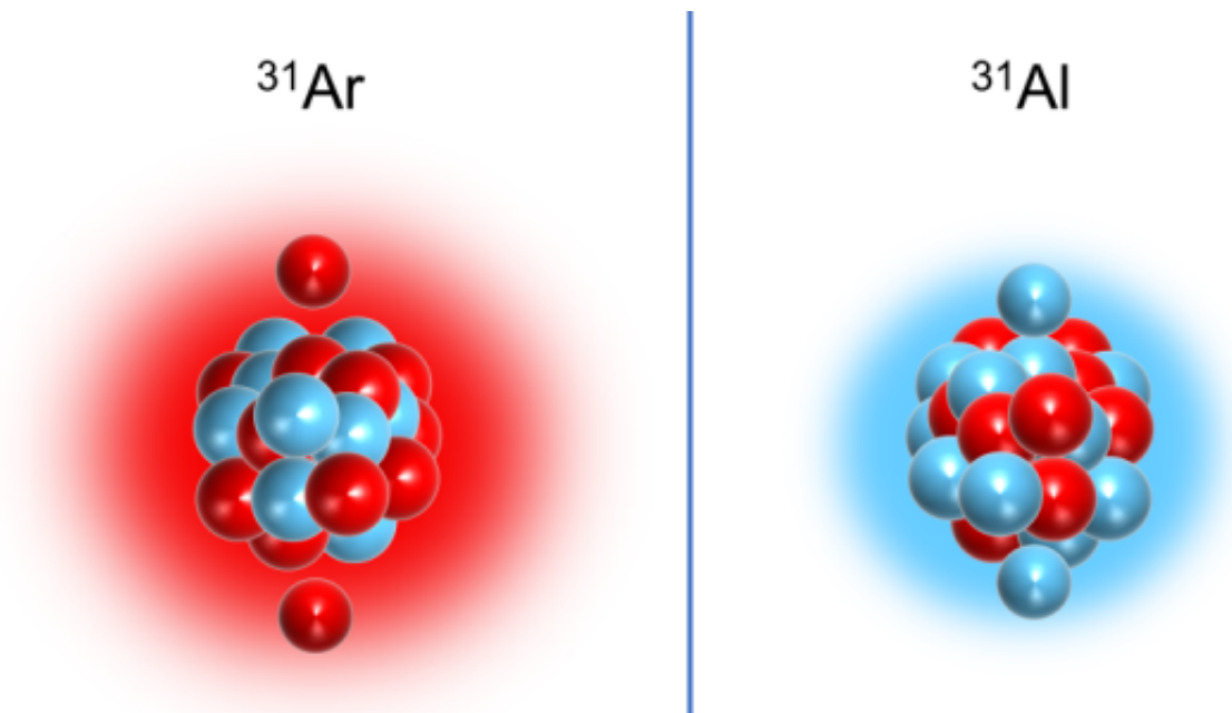
镜像核氩-31和铝-31的核子分布示意
