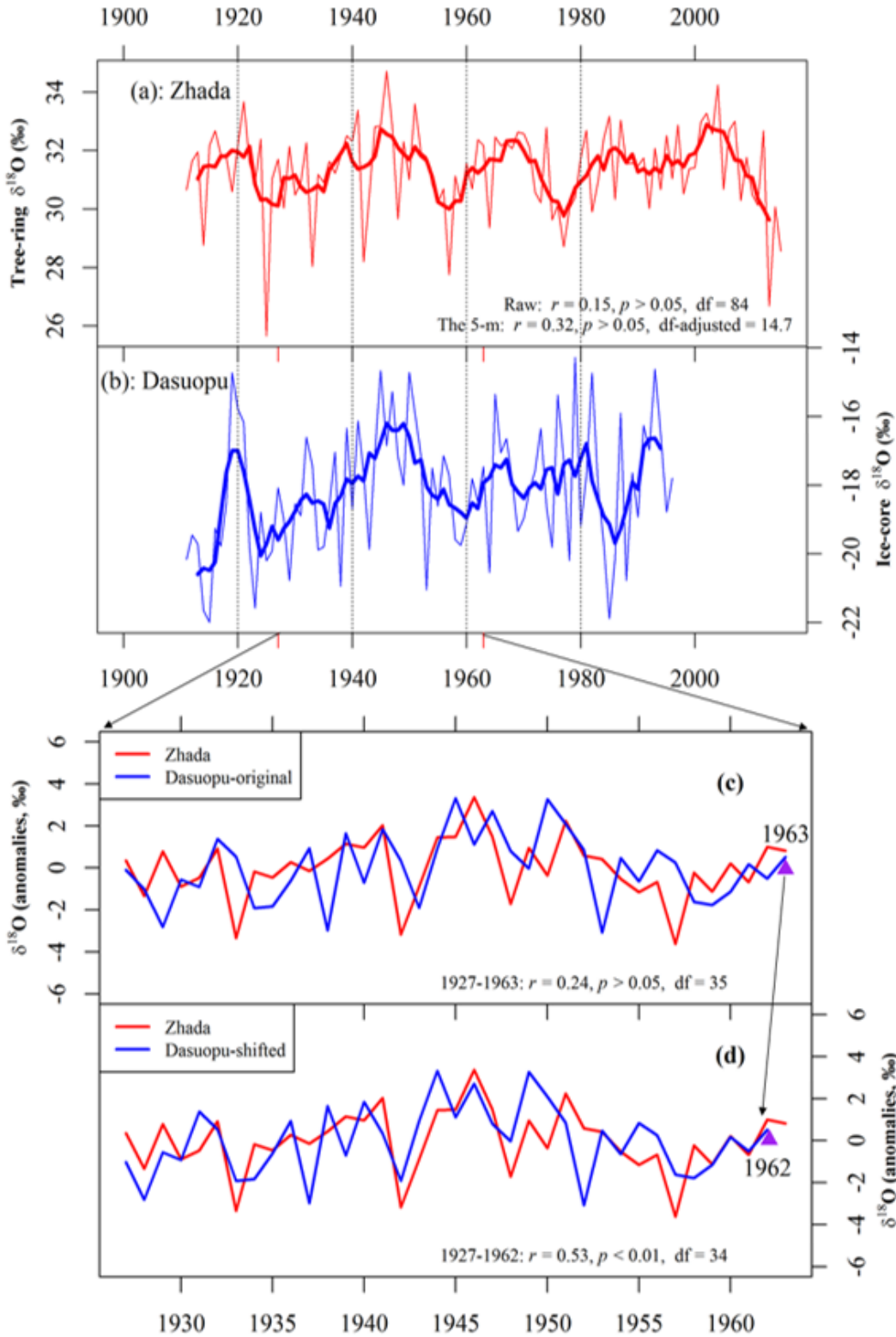
图4. 札达树轮氧同位素(红线)与达索普冰芯氧同位素(蓝线)的对比。(a)和(b)中的细线、粗线分别表示年值和5年滑动值。(c)和(d)为树轮氧同位素和达索普冰芯氧同位素的对比，(d)展示了冰芯标志年调整为1962之后，二者匹配更为一致。
