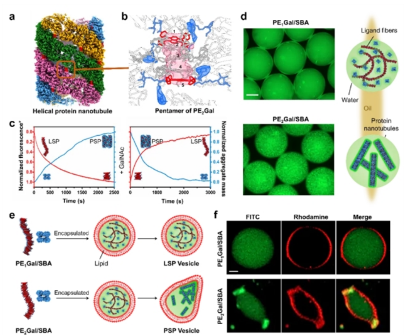
图2：牺牲型超分子聚合物诱导的人工蛋白微管形成。
