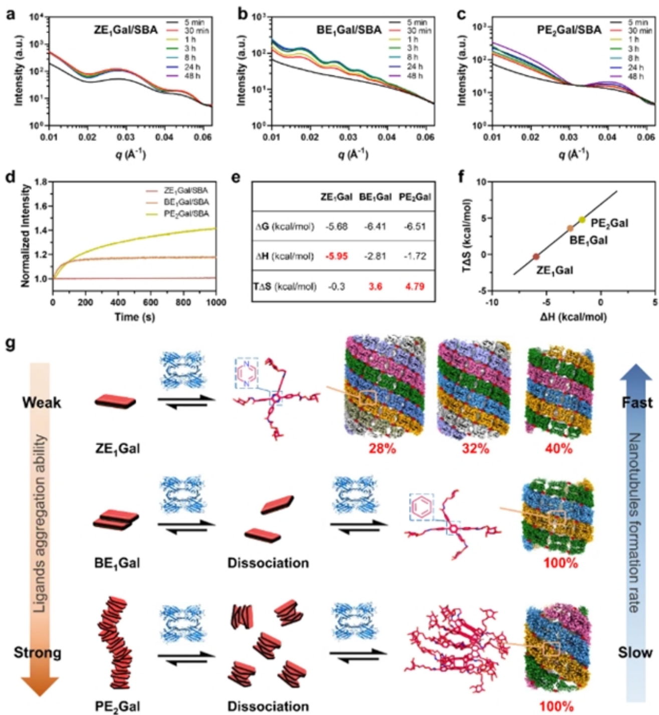
图4：人工蛋白微管形成的动力学和热力学特征。
