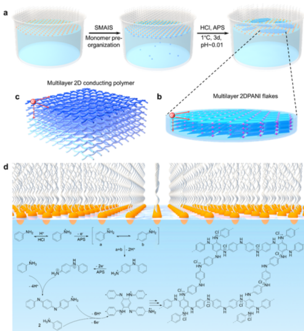
二维聚苯胺结构及制备过程示意图
