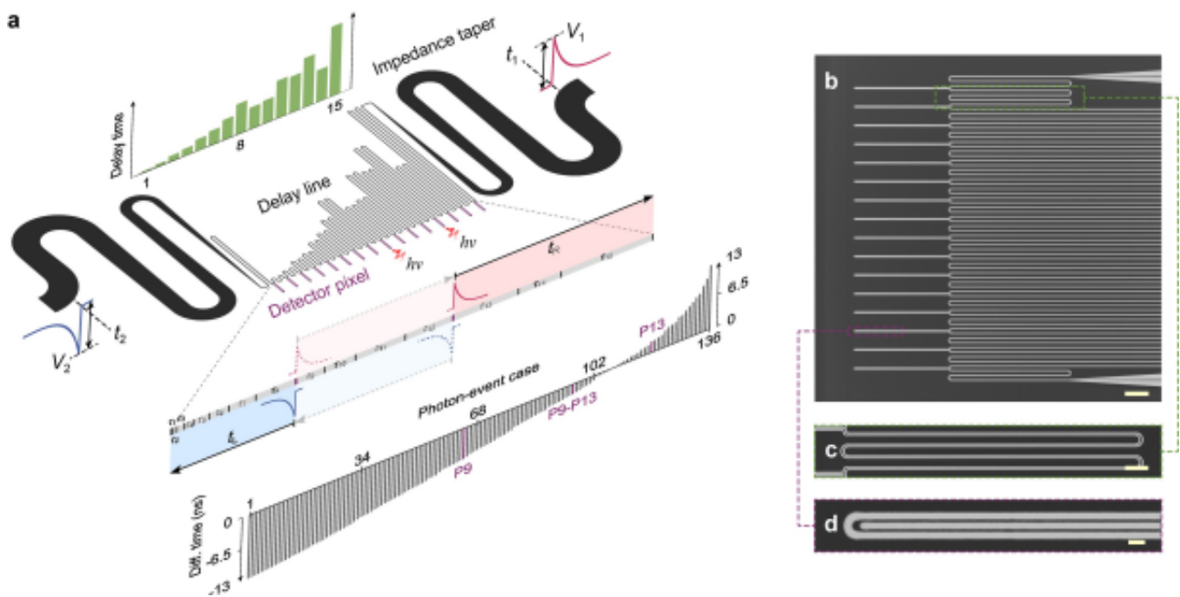
16单元器件的结构示意图和电子显微图
