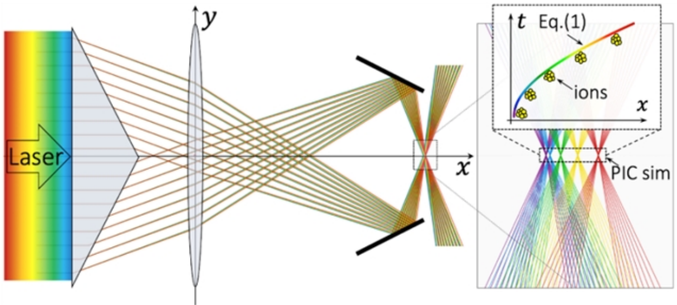
图 1：慢速激光离子加速的方案示意图
