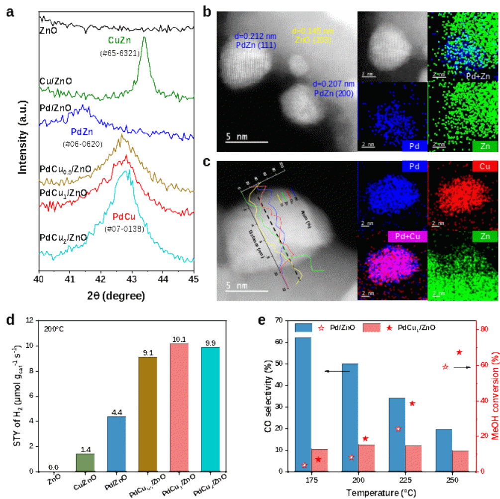
PdCu x /ZnO催化剂的（a）晶体结构、（b、c）微观形貌、MSR反应的（d）氢气产率、（e）CO选择性和甲醇转化率
