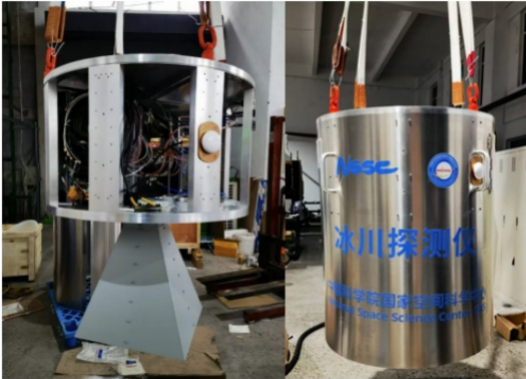
机载超宽带高光谱微波辐射计实物
