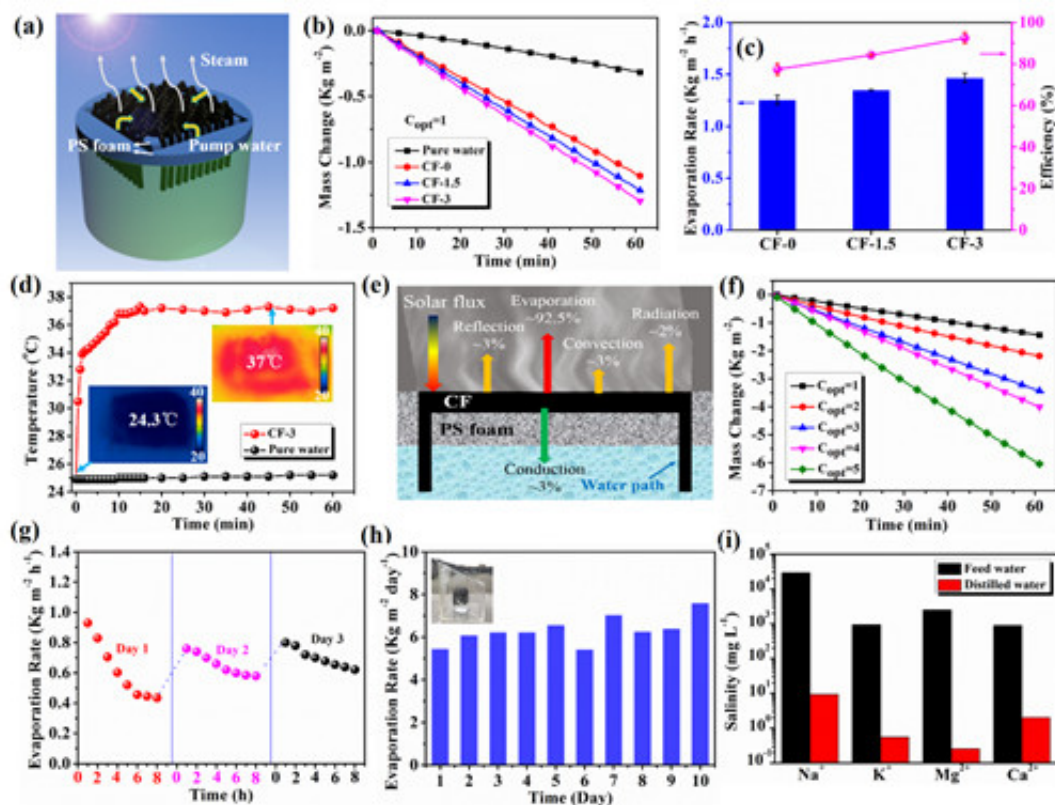
图1 碳化改性碳纤维光热转化性能
