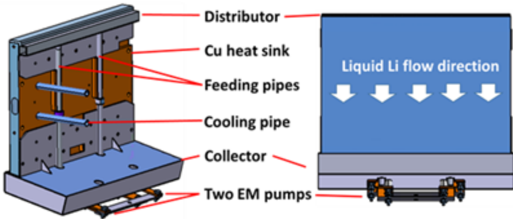
图1 二代流动液态锂限制器结构示意图
