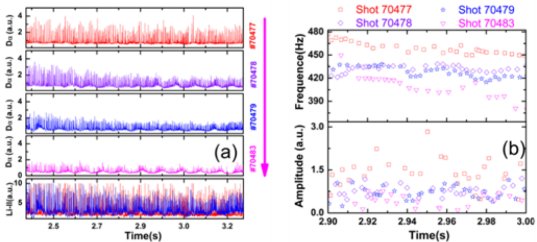
图3 流动液态锂壁条件下ELM行为变化：随着放电的持续ELM逐渐缓解(a)，ELM的频率与幅值(b)
