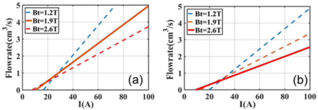
图2 双电磁泵(a)和单电磁泵(b)条件下锂的流量与电磁泵电流的关系
