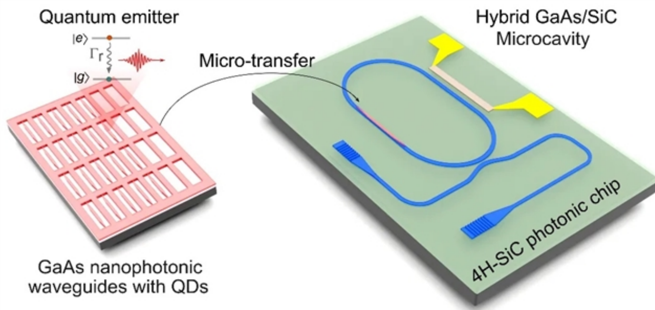
图1：基于III-V量子点和电光4H-SiC材料的混合集成量子点微腔
