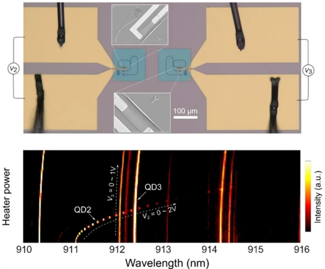
图3：片上可扩展微腔耦合量子点光源
