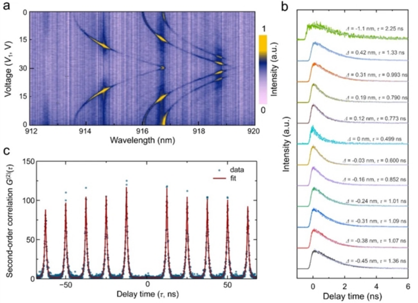
图2：（a）片上调控微腔耦合量子点单光子信号；（b）量子点荧光增强；（c）片上微腔增强量子点单光子纯度测试
