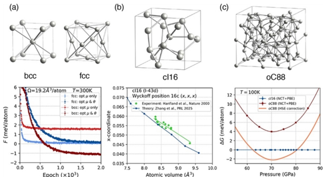
图. (a) 低压下，锂的 bcc-fcc 结构转变起源于非简谐核量子效应所引起的自由能反转；(b) 50GPa附近cl16 结构中计算预测的锂原子分数坐标与实验观测数据的对比；(c) 70GPa附近实验所观察到的oC88结构起源于高精度密度泛函理论对自由能的修正。
