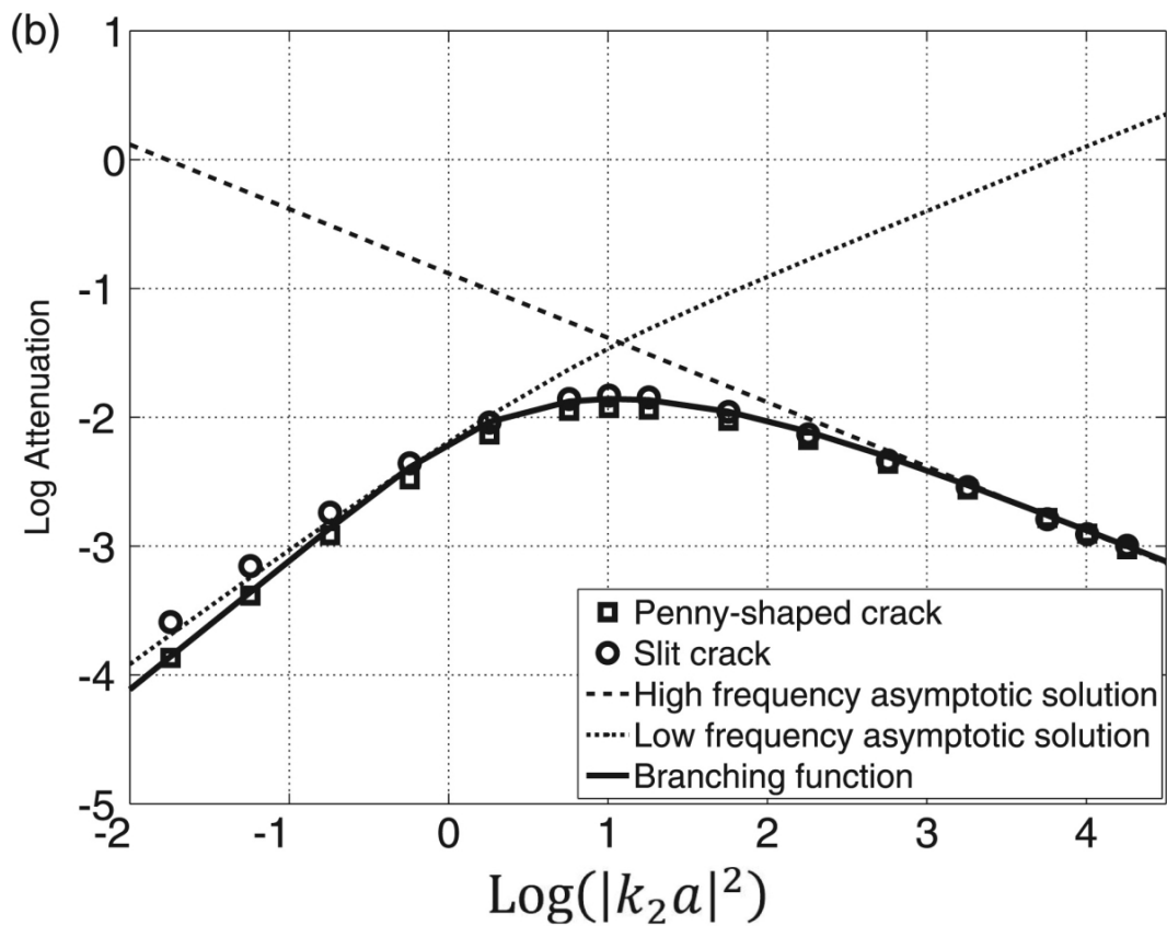
图2 不同模型计算值对比(a)速度频散对比;(b)能量衰减对比
