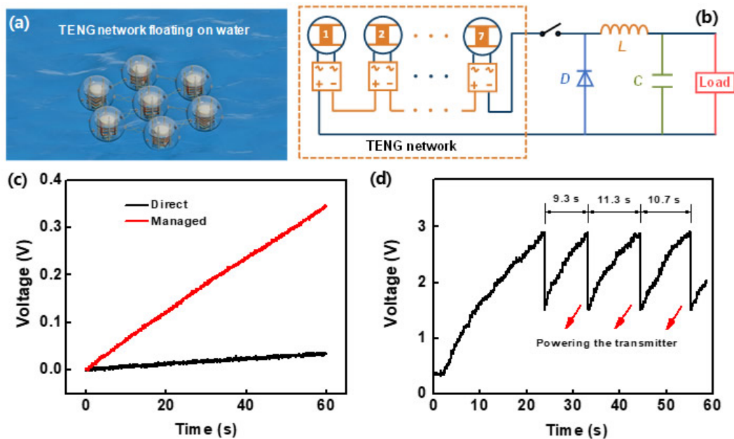
(a)球形摩擦纳米发电机网络的结构示意图;(b)海洋能摩擦纳米发电网络能量管理的原理示意图;(c)给10mF电容器直接充电与能量管理后充电的电压曲线比较;(d)能量管理后的发电机网络驱动无线发射器时的电压曲线。
