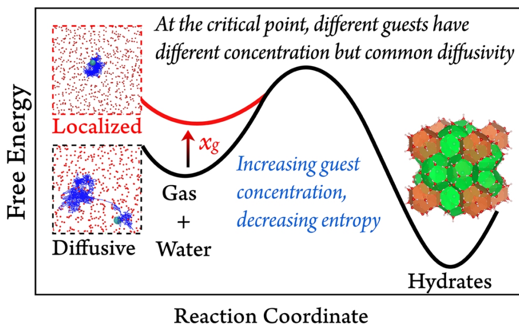
图2随着溶液中气体分子浓度( x_g )的增大，体系总熵降低，自由能增加，气体分子的扩散系数趋近于一个临界值
