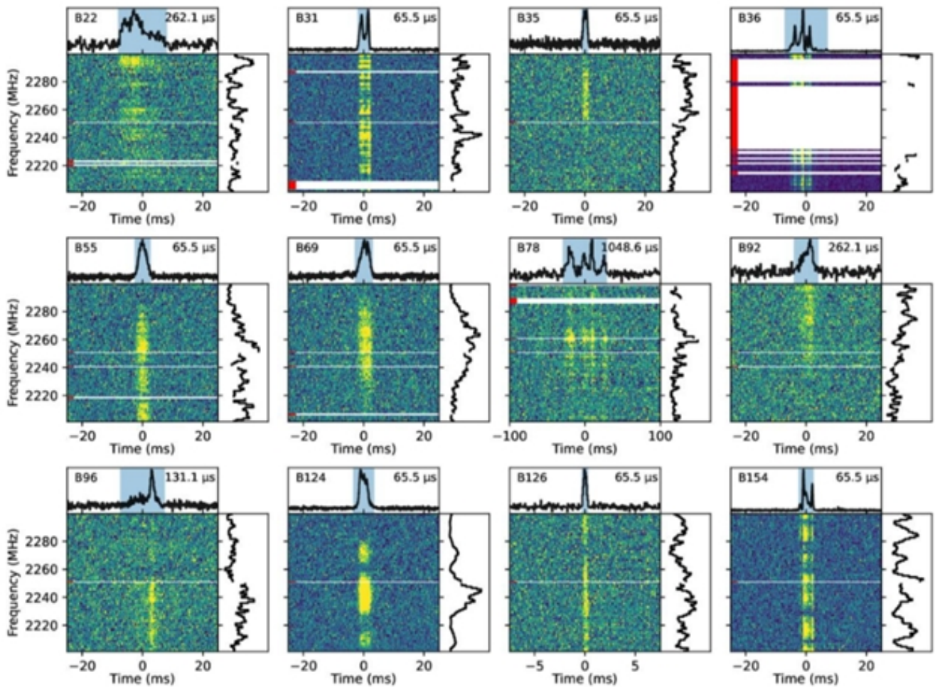
天马探测到的FRB 20240114A部分爆发示意图
