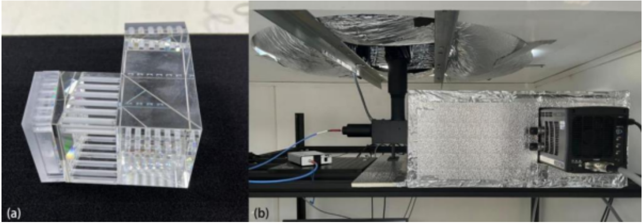
(a) 一体化ASHS干涉模块，(b) 野外观测站的ASHS干涉仪配置
