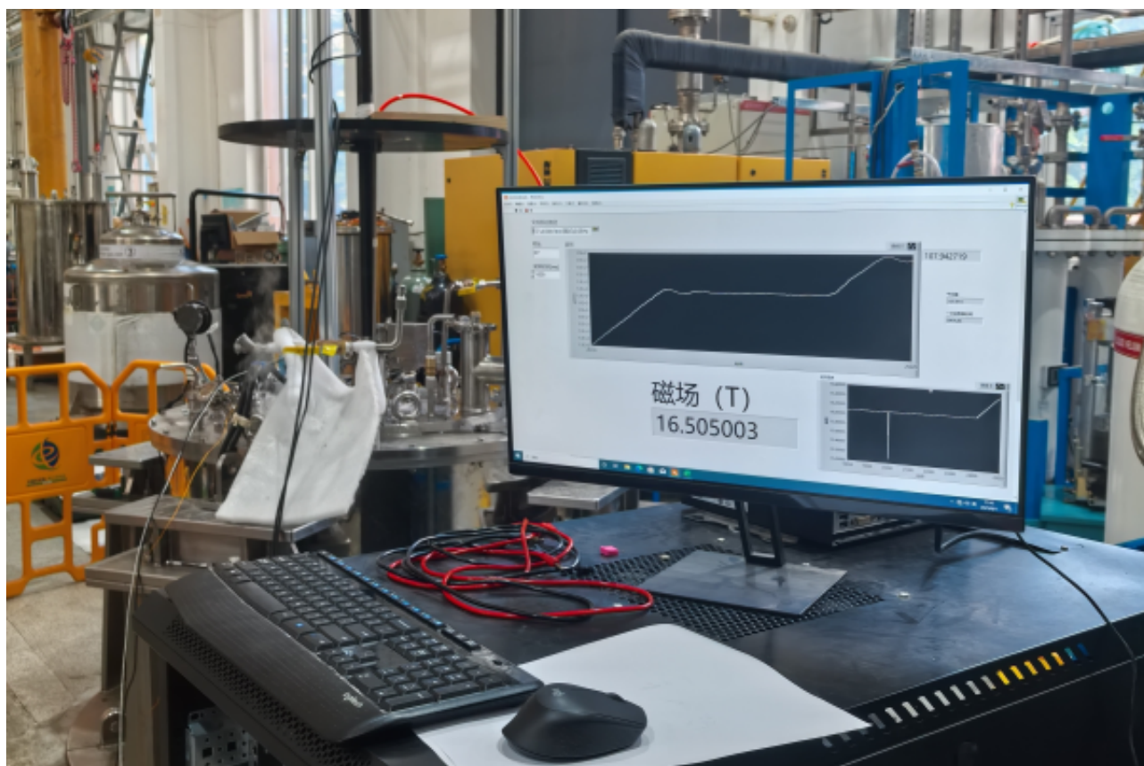
大口径高场超导磁体测试现场
