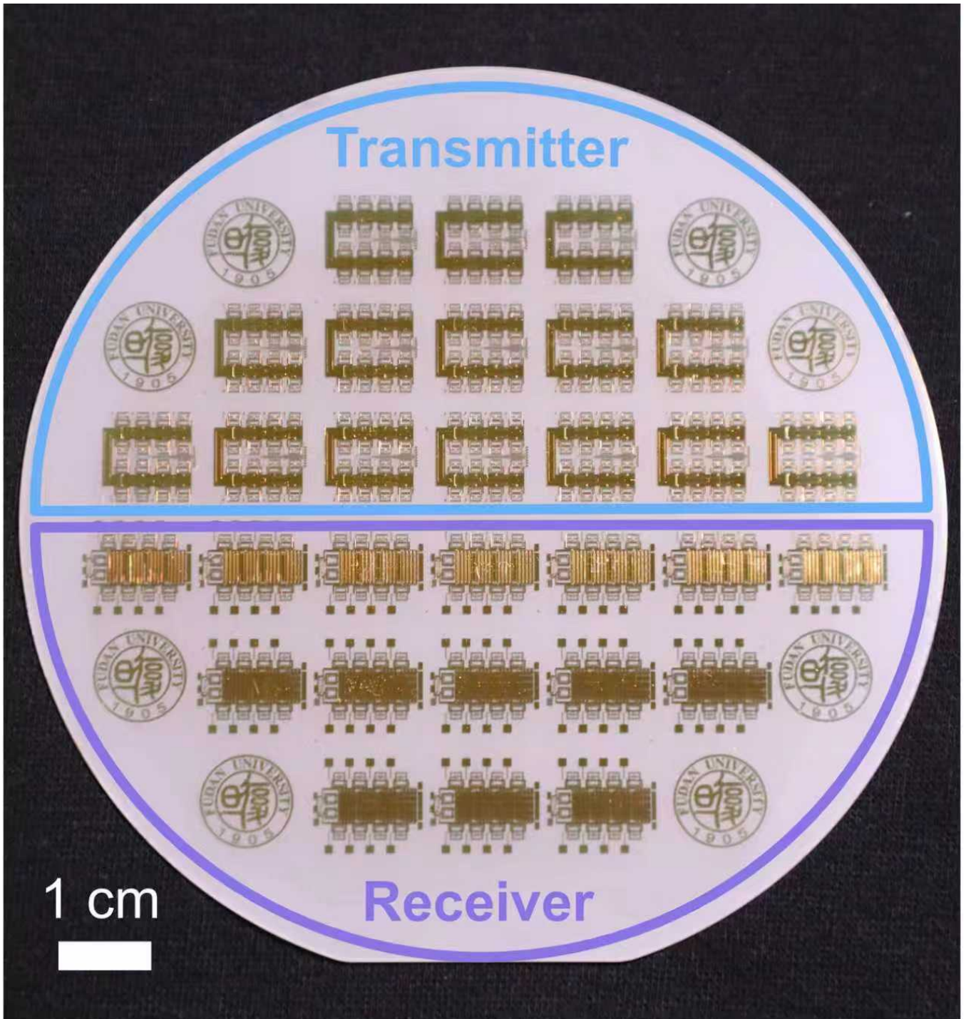
4英寸原子层半导体抗辐射射频通信芯片。研发团队供图
