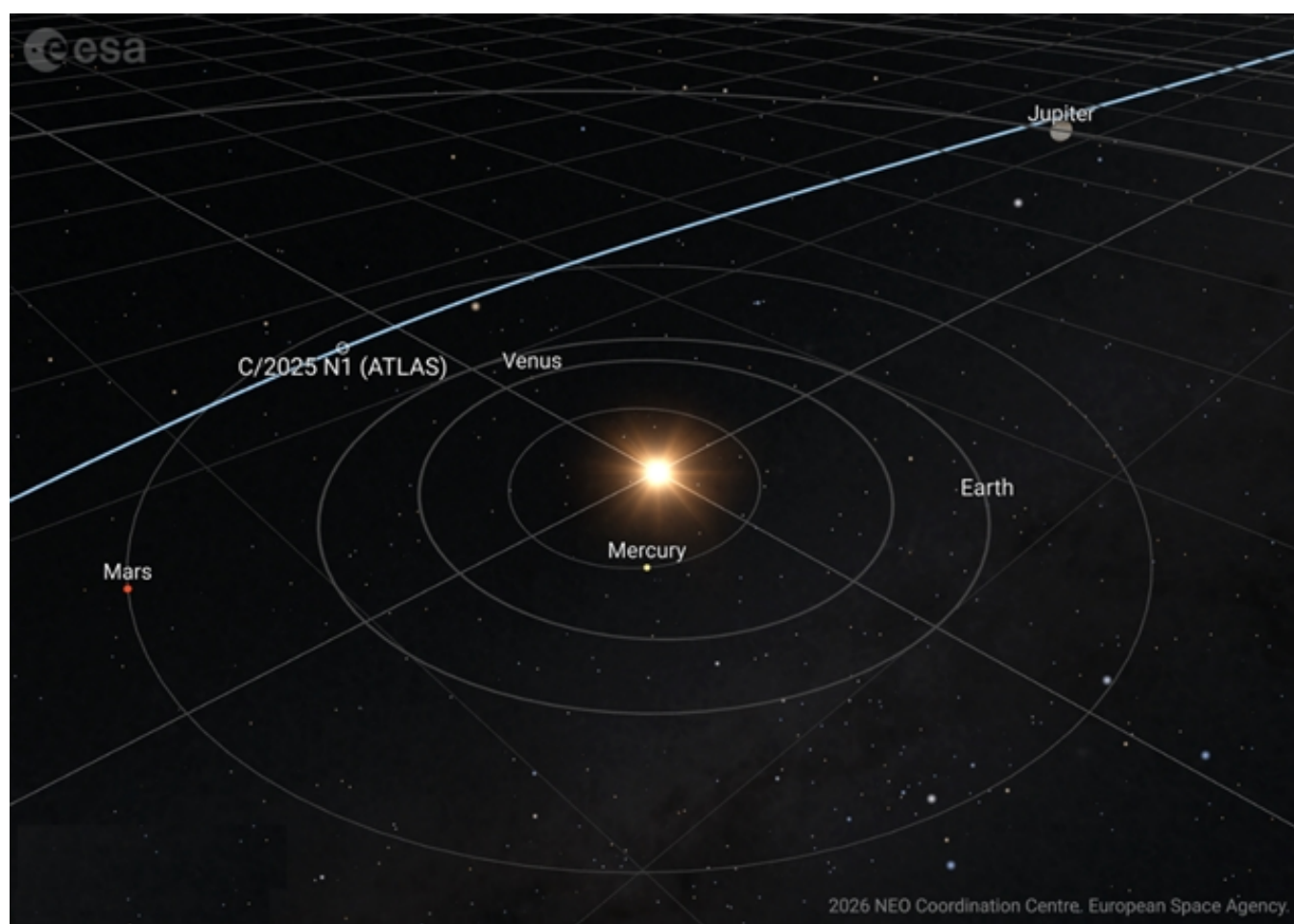
彗星3I/ATLAS穿越太阳系内侧的轨迹示意图。来源：ESA NEOCC
