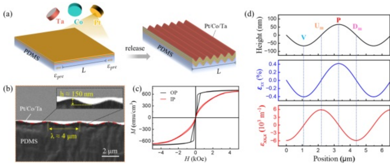
褶皱Pt/Co/Ta多层膜的制备、形貌、磁性表征与应变分布
