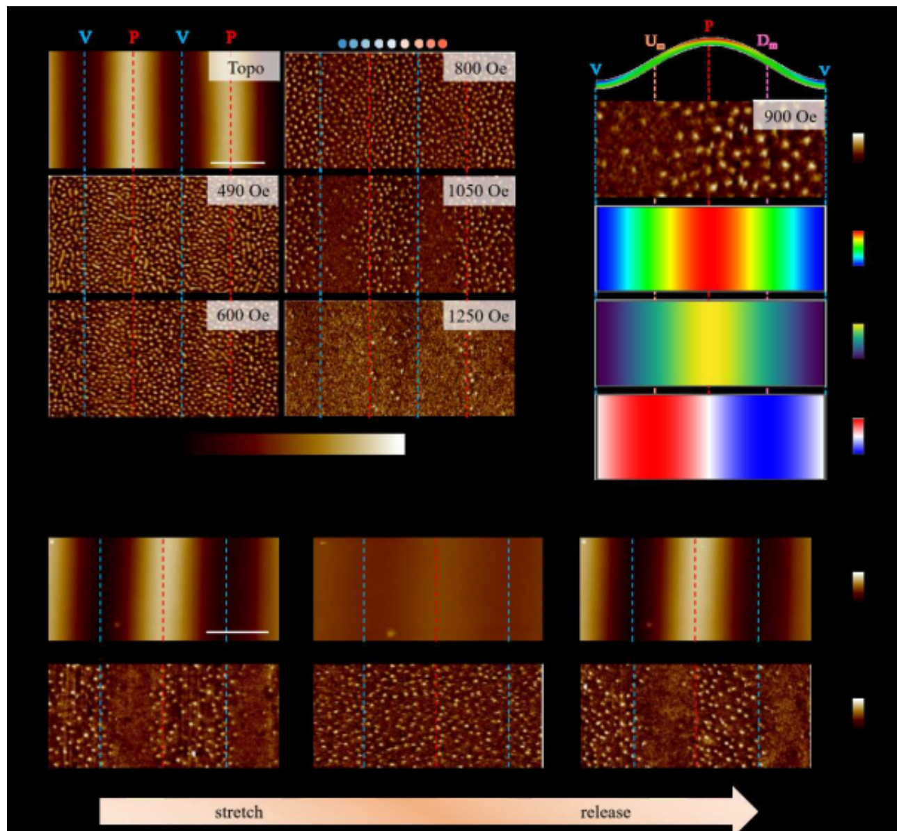
褶皱Pt/Co/Ta多层膜的制备、形貌、磁性表征与应变分布
