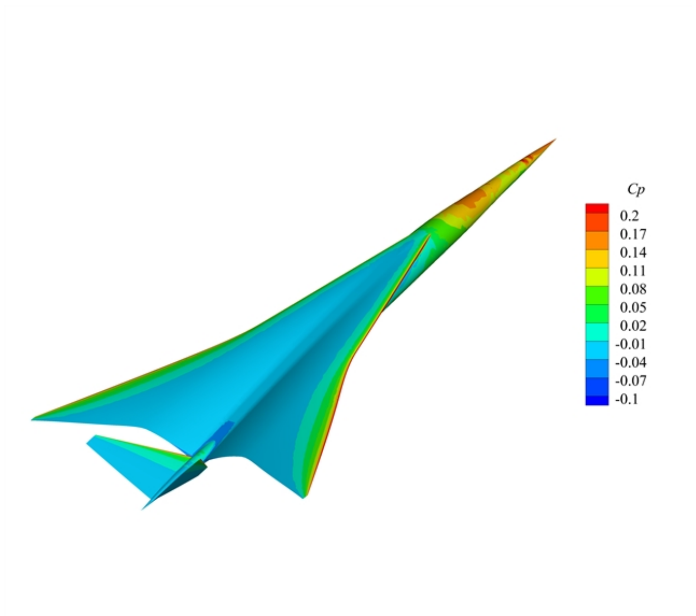
超声速民机表面压力系数云图
