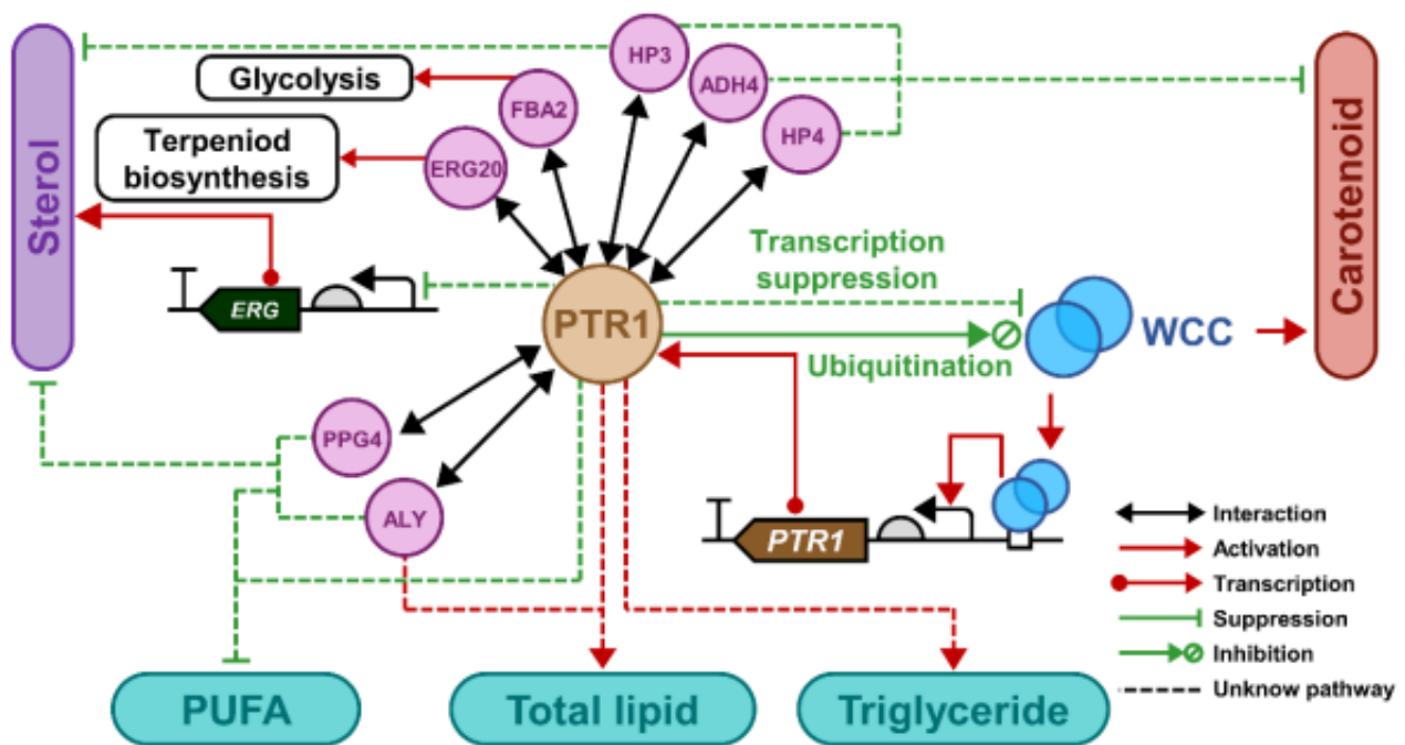
PTR1调控类胡萝卜素、甾醇和脂质代谢的模型
