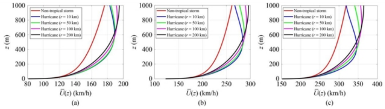
图2.墨西哥坎昆10分钟平均时距下的平均风速：非热带风暴与登陆飓风对比: (a) 10年一遇风； (b) 50年一遇风； (c) 200年一遇风。
