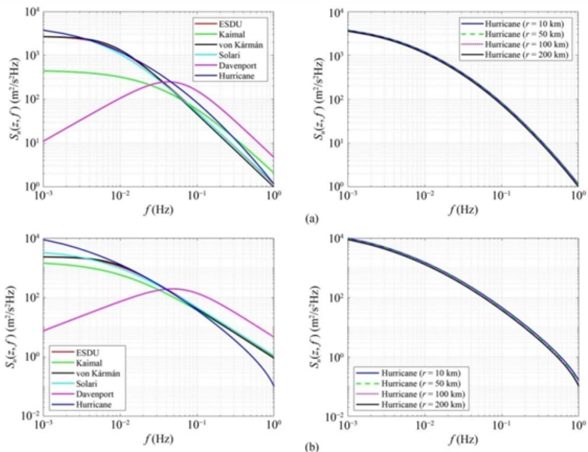
图3.墨西哥坎昆200年一遇风在10分钟平均时距下的功率谱密度函数: (a) z=10\text{m} 处非热带风暴与登陆飓风对比; (b) z=200\text{m} 处非热带风暴与登陆飓风对比。
