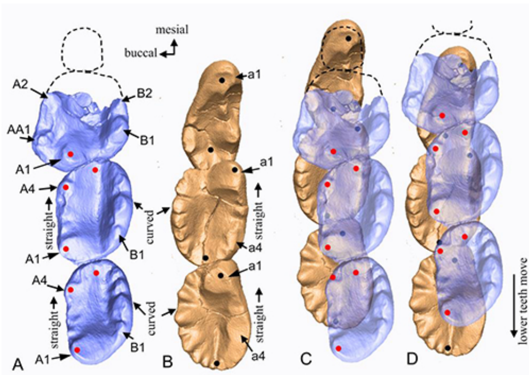
济赞堂奇兽牙齿磨痕的SEM显微结构，显示磨蚀面、磨痕及其分布(毛方圆 供图)
