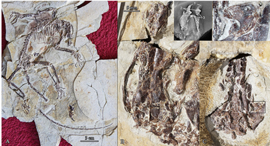
济赞堂奇兽模式标本以及头骨、外鼓骨形态(毛方圆 供图)
