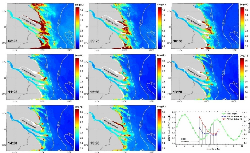
图：遥感反演的2016年3月1日长江口表层POC浓度。利用GOCI影像，可以反演每天八个时刻的表层POC浓度。右下图展示的是长江口徐六泾(S1)和北支口门(S2)的时间序列POC浓度及潮高
