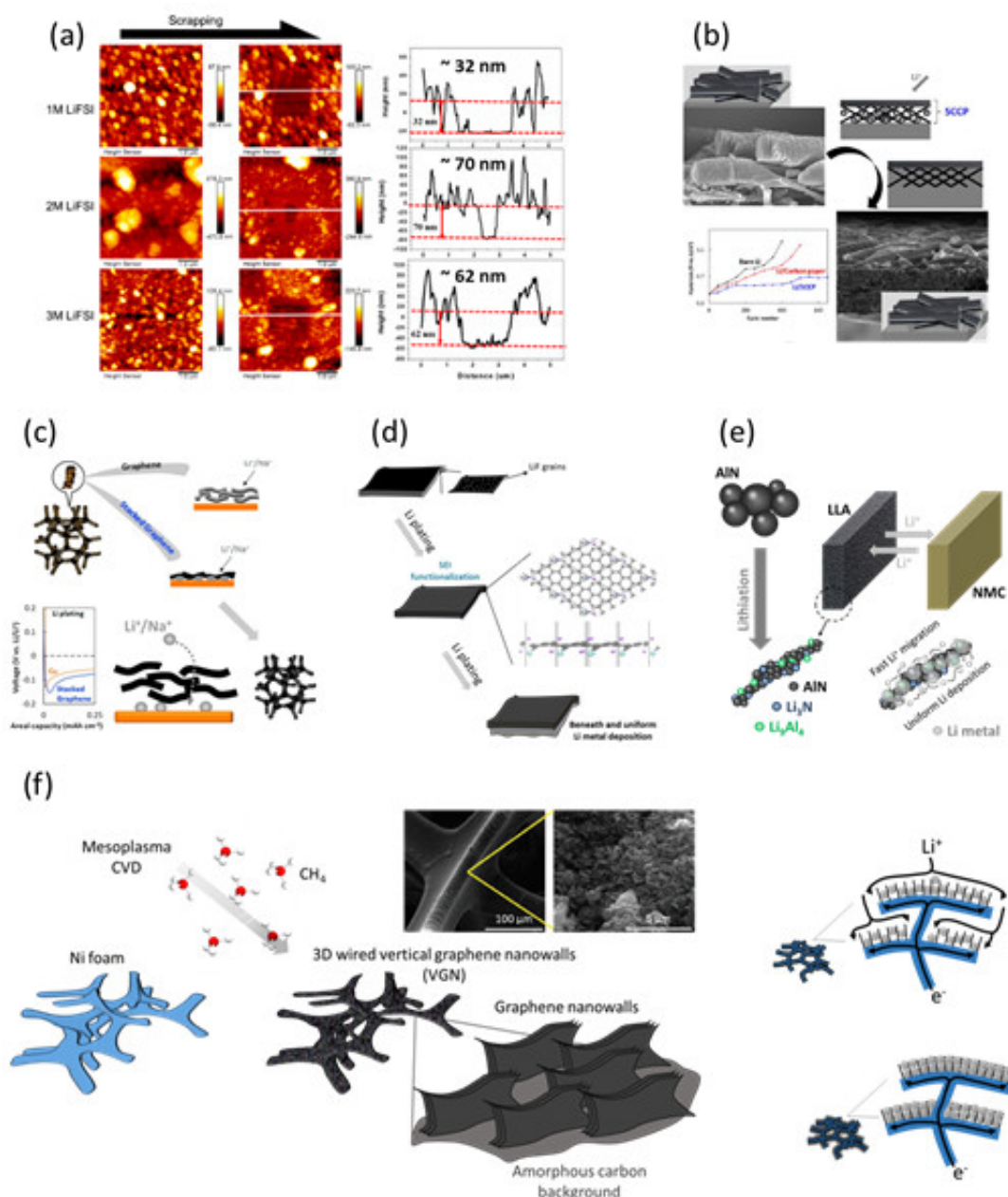
图1(a)锂金属负极界面在不同盐浓度下的界面表征;(b)一种用于锂金属界面保护的导向性双层碳结构;(c)一种堆叠石墨烯实现的过滤型锂金属沉积保护模式;(d)一种碳缺陷位点的界面转化实现SEI化的功能性锂金属保护层;(e)一种简易制备的Li 9 Al 4 -Li 3 N-AlN结构作为高效的锂金属宿主结构;(f)一种垂直石墨烯结构实现的特殊界面锂离子传输及锂金属均匀沉积。
