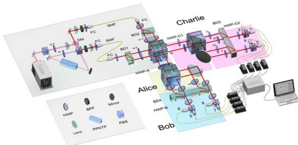
Bell基测量的自检验实验装置
