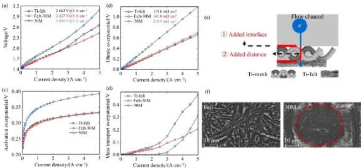
图5.PEM水电解中钛毡、钛网及堆叠梯度PTL的电化学性能对比与界面接触效应。
