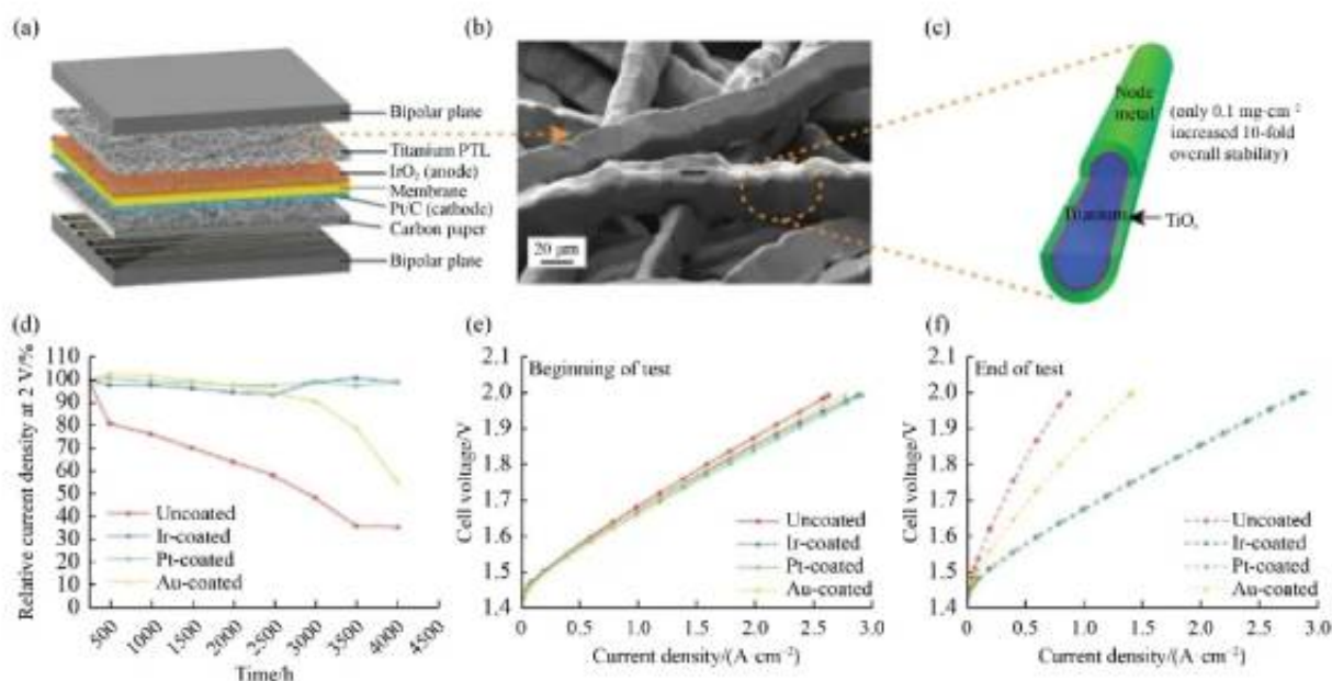
图7.超薄贵金属涂层钛纤维PTL的结构与电化学性能。
