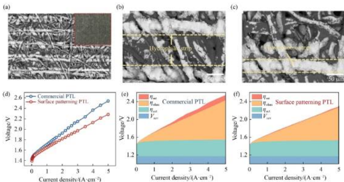
图6.PEM水电解中双亲图案化钛毡PTL的表面表征与电化学性能分析。
