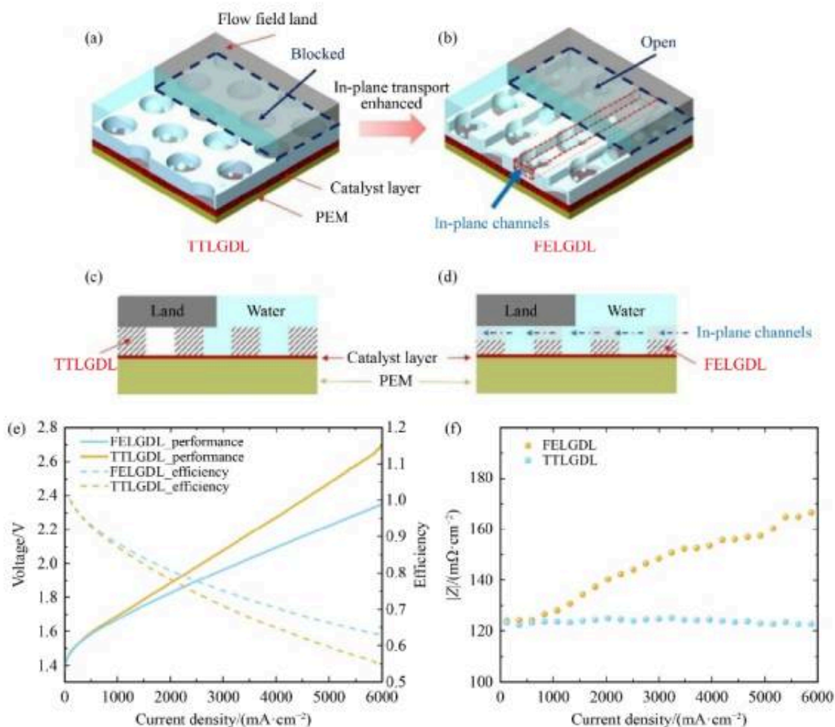
图4.二维与三维结构化PTL的设计示意图及PEM水电解中两相传输性能对比。
