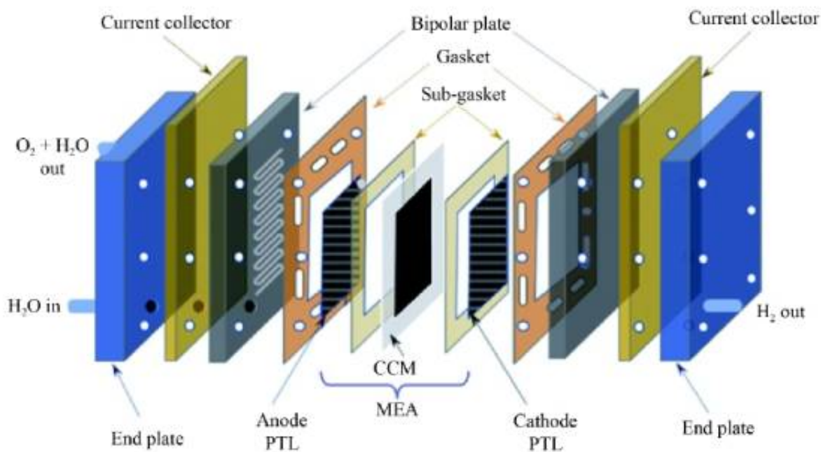
图2.典型PEMWE单电池的分解视图，突出显示PTL作为关键功能部件。
