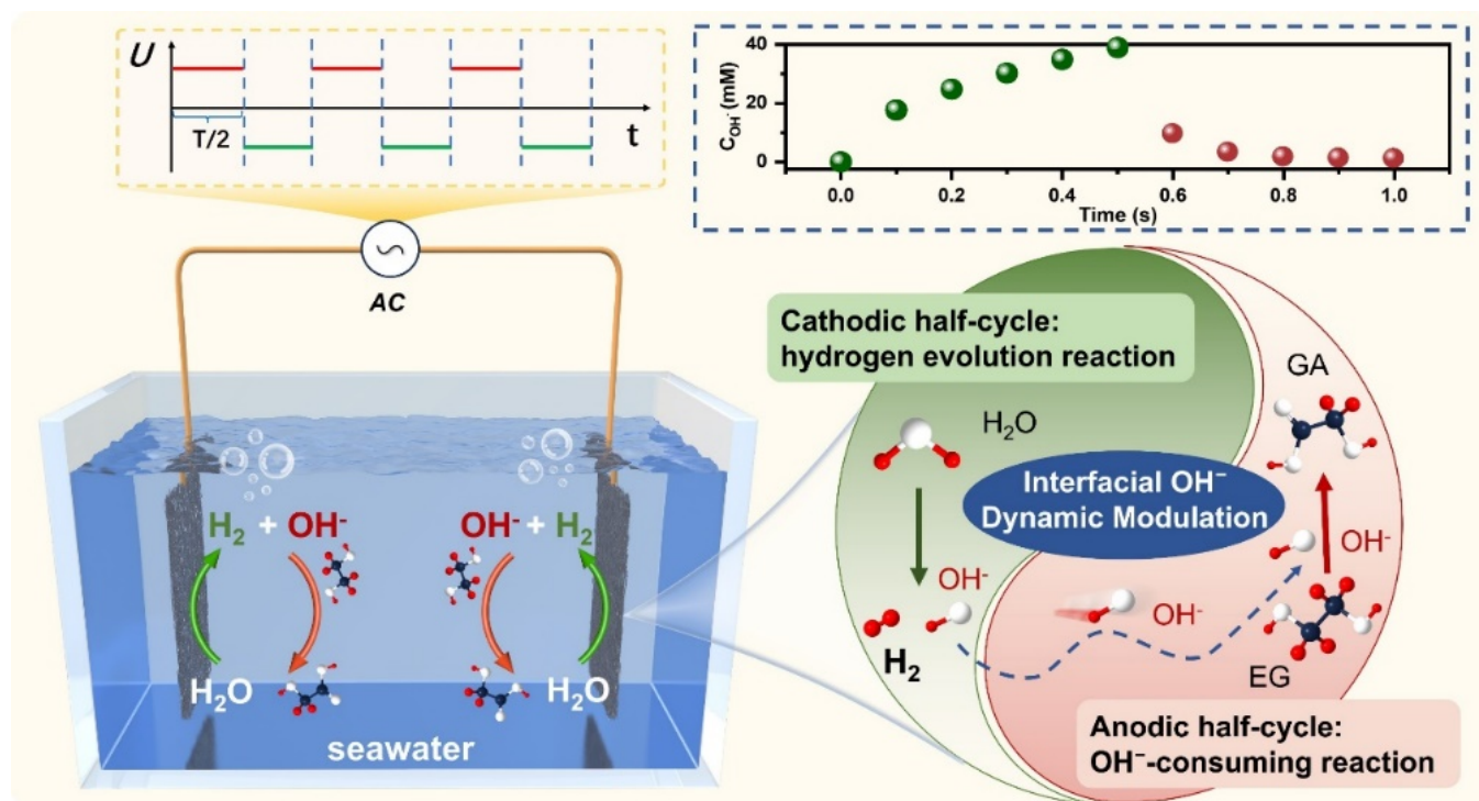
交流电直接海水电解制氢原理示意图。理化所供图
