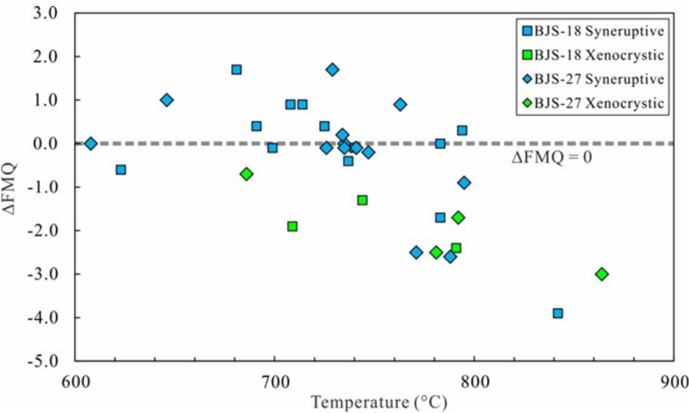
图4 来自样品 BJS-18 和 BJS-27 的同喷发锆石与捕获锆石的温度—氧逸度关系图。温度采用锆石钛
