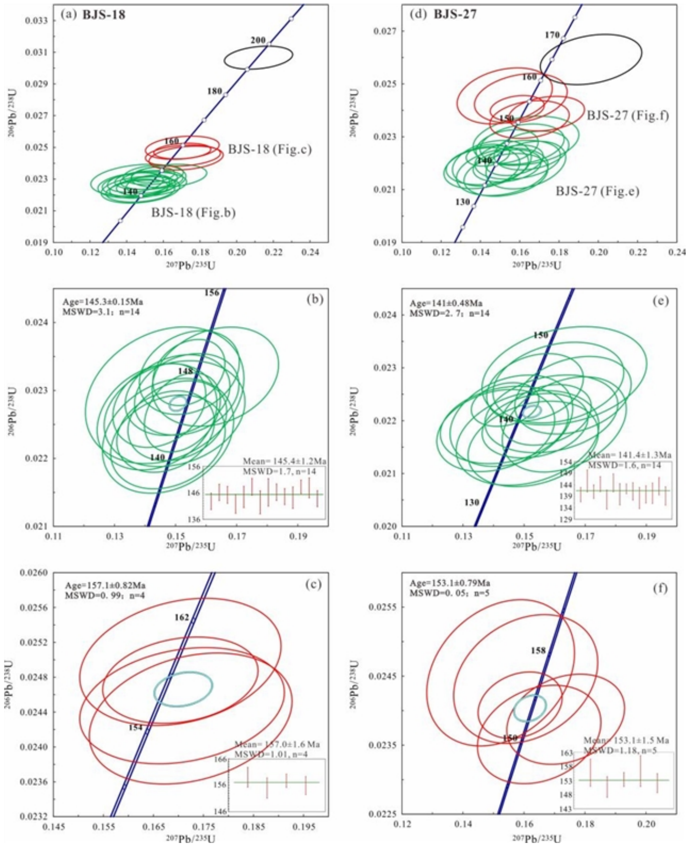
图2. 笔架山火山岩锆石U - Pb谐和图及加权平均年龄
