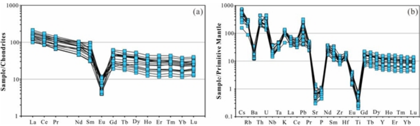
图3 笔架山火山岩全岩稀土、微量元素特征
