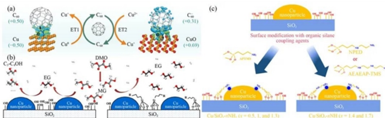
图3.C60与硅烷偶联剂修饰铜基催化剂（图8），通过电子转移效应稳定Cu + 价态，抑制其向Cu 0 或Cu 2+ 转化，有效解决了催化剂易失活的问题。
