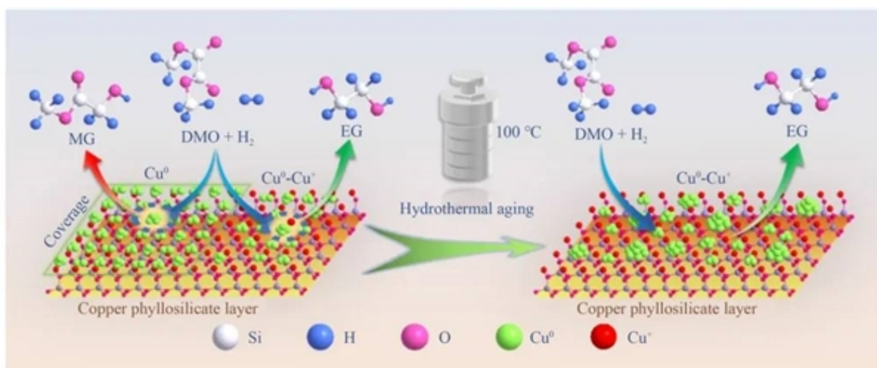
图2.水热老化调控Cu-SiO 2 催化剂（图5），优化了Cu + 在铜层状硅酸盐层间的分散性，进一步强化Cu + 与Cu 0 的协同作用，显著提升EG合成效率。
