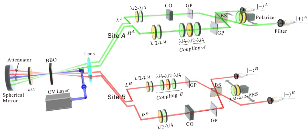
实现非局域可观测量的量子测量的实验装置图
