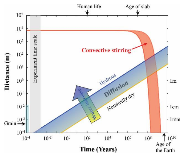
图：利用扩散系数估算的地幔过渡带内俯冲板块的均一化程度与地幔过渡带可能的含水量
