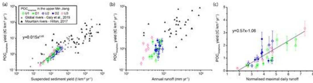
图2 生物有机碳侵蚀速率和物理侵蚀速率、径流量、最大日径流量的关系
