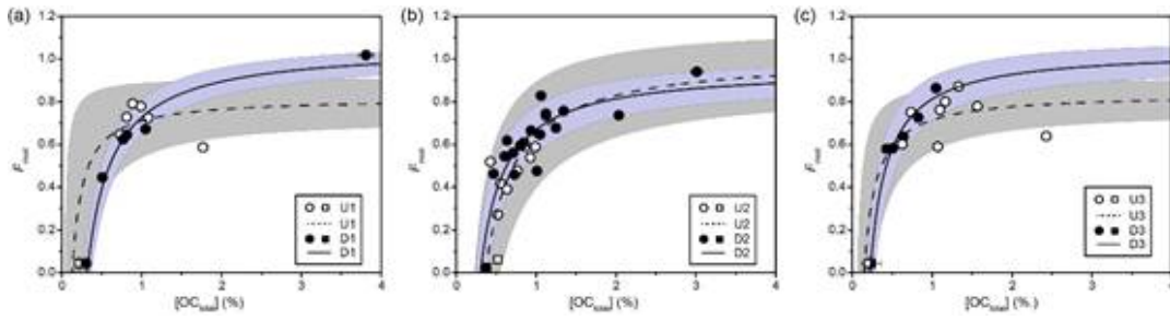
图1 利用有机碳含量及 14 C同位素计算各个站点的化石有机碳含量和生物有机碳年龄
