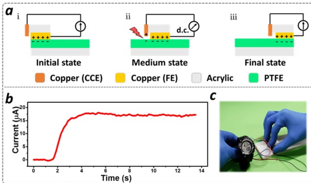
图：(a)恒流摩擦纳米发电机的工作原理，(b)该TENG的恒电流输出，(c)该TENG直接驱动电子手表(无整流和储能单元)。
