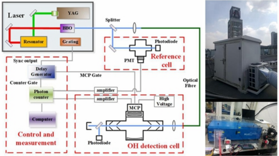
图1 OH自由基激光诱导荧光探测系统的原理图和实物图
