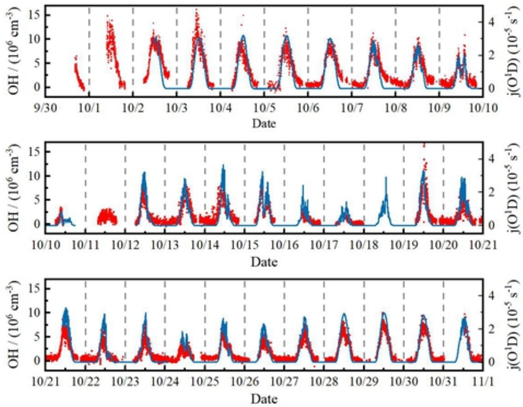
图2 STORM期间的OH和j(O1D)时间序列
