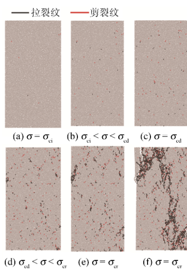
图2岩石单轴压缩破坏过程微裂纹分布及微裂纹增长曲线
