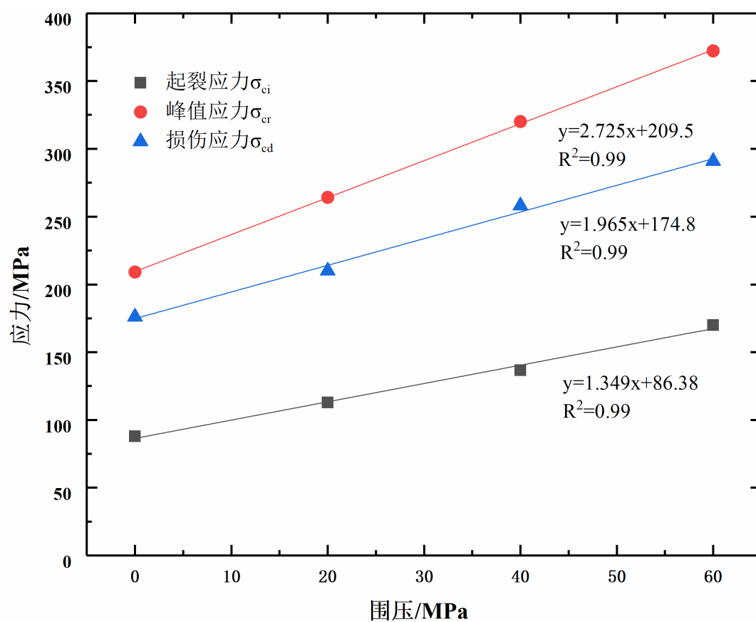
图3 不同应力条件岩石特征应力
