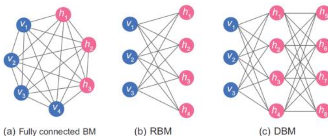
三种玻尔兹曼机示意图：(a)全连接玻尔兹曼机；(b)受限玻尔兹曼机；(c)深度玻尔兹曼机。
