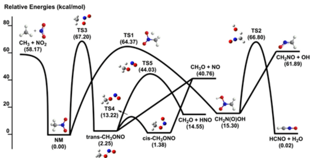
图1 硝基甲烷在0K时分解的势能面
