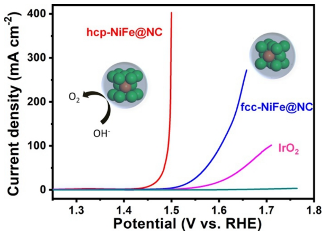
图：不同晶体结构NiFe合金与贵金属基催化剂的析氧反应极化曲线对比。
