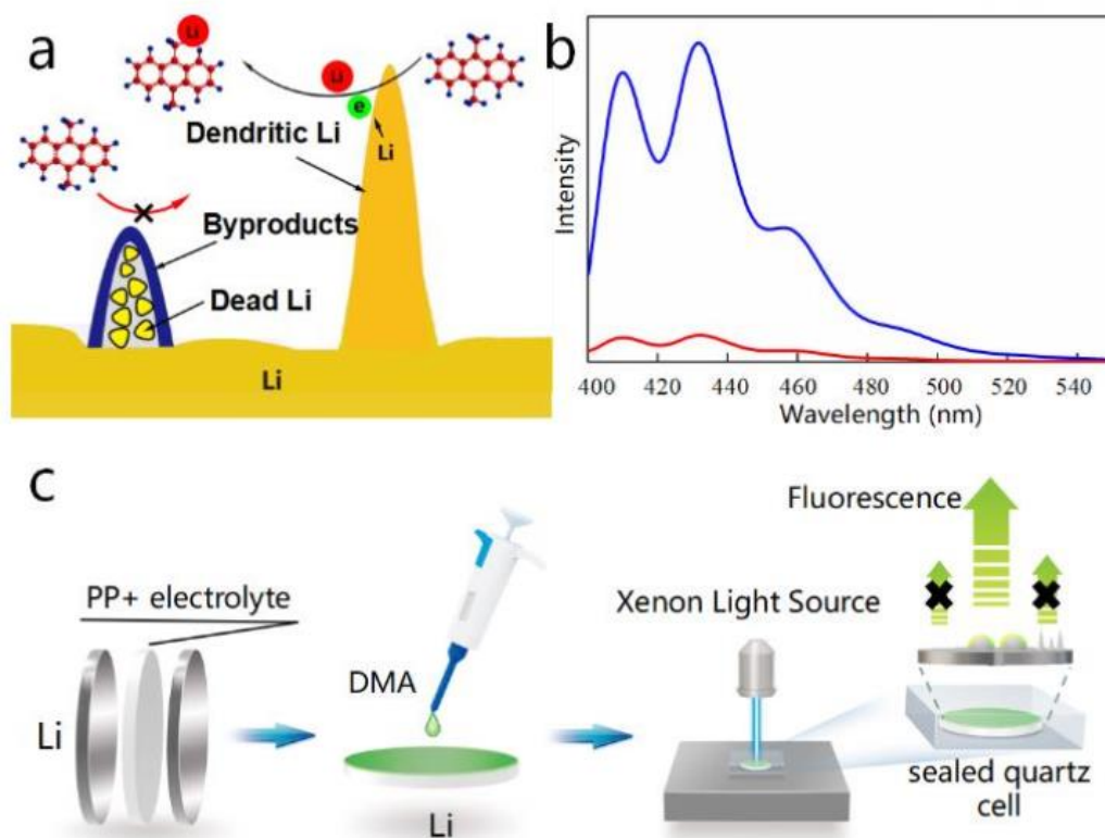
(a)DMA与锂金属表面成分反应示意图;(b)TEGDME/DME(1:1)中5 mg mL -1 的DMA被金属锂处理前后(蓝线为处理前，红线为处理后)的发射光谱曲线;(c)DMA探针法观察循环后锂金属表面活性锂分布的过程
