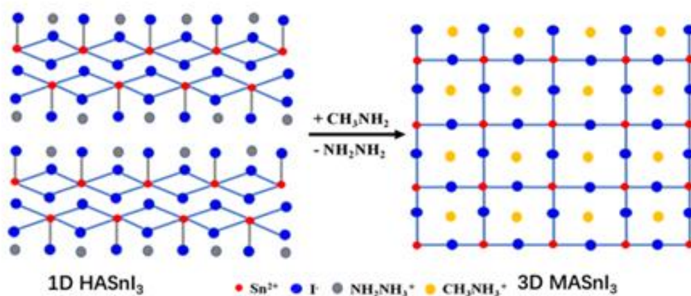
图2 从1D到3D—固气反应制备锡钙钛矿( \text{CH}_3\text{NH}_3\text{PbI}_3 )薄膜
