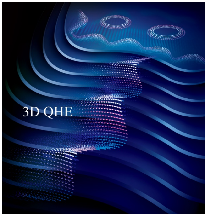
图1：三维量子霍尔效应及电荷密度波示意图。由于磁场效应，体内电子在面内的运动形成朗道能级，如上方圆圈所示。在仅有一个Landau能级被占据的量子极限下，更强的电子关联效应导致电荷密度波的形成，并进而使得体系转化为三维量子霍尔绝缘体。
