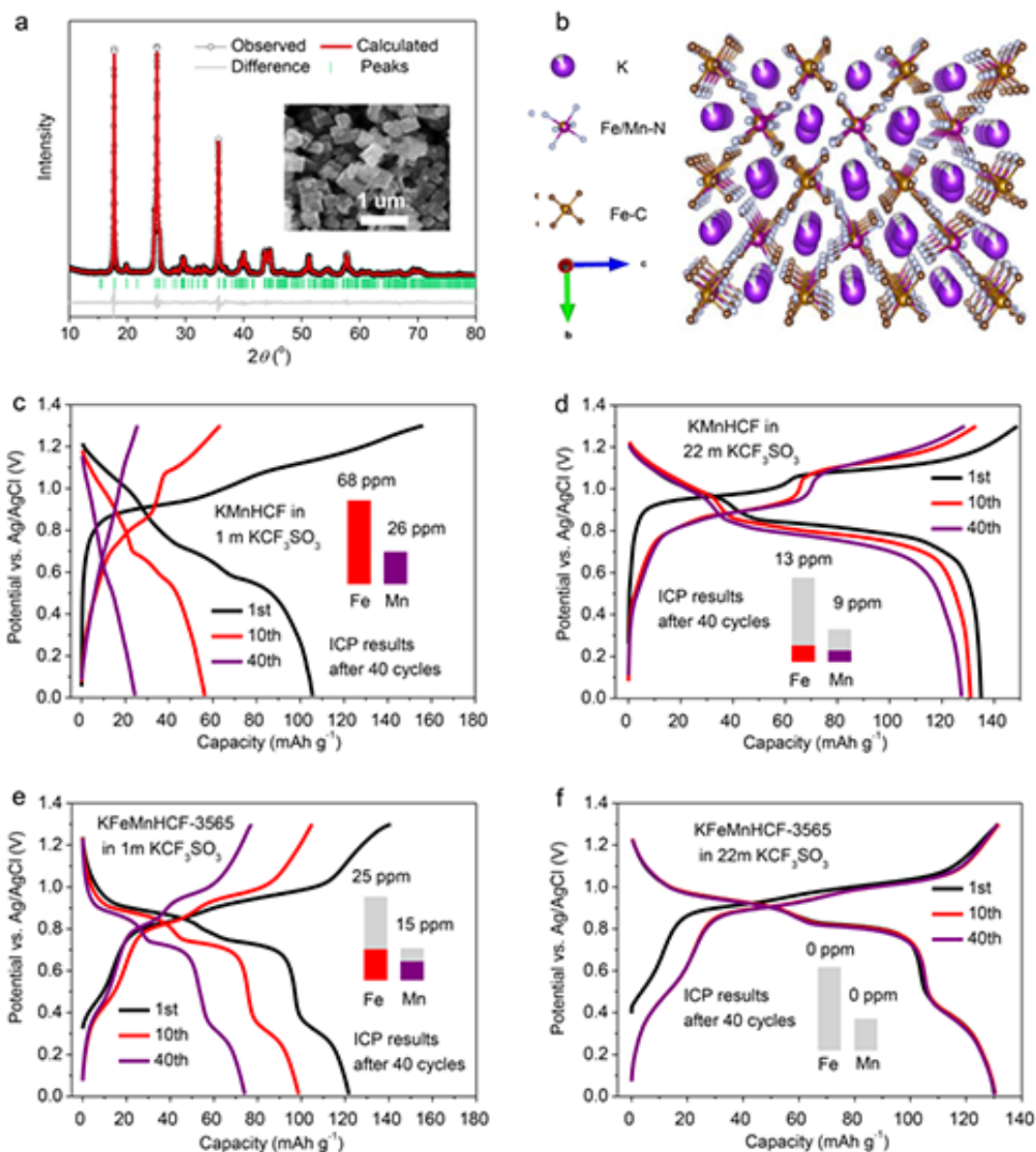
图1. Fe取代富锰普鲁士蓝正极材料的结构与性能优化。(a)Fe取代的KFeMnHCF-3565正极材料的XRD精修图;(b)具有P21/n空间群的 \text{K}_x\text{Fe}_z\text{Mn}_{1-y}[\text{Fe}(\text{CN})_6]_w \cdot z\text{H}_2\text{O} 典型结构图;(c-f)无取代材料(KMnHCF)和有Fe取代的材料(KFeMnHCF-3565)在1mol/L和22mol/L三氟甲基磺酸钾电解液中的电化学以及过渡金属溶解情况。
