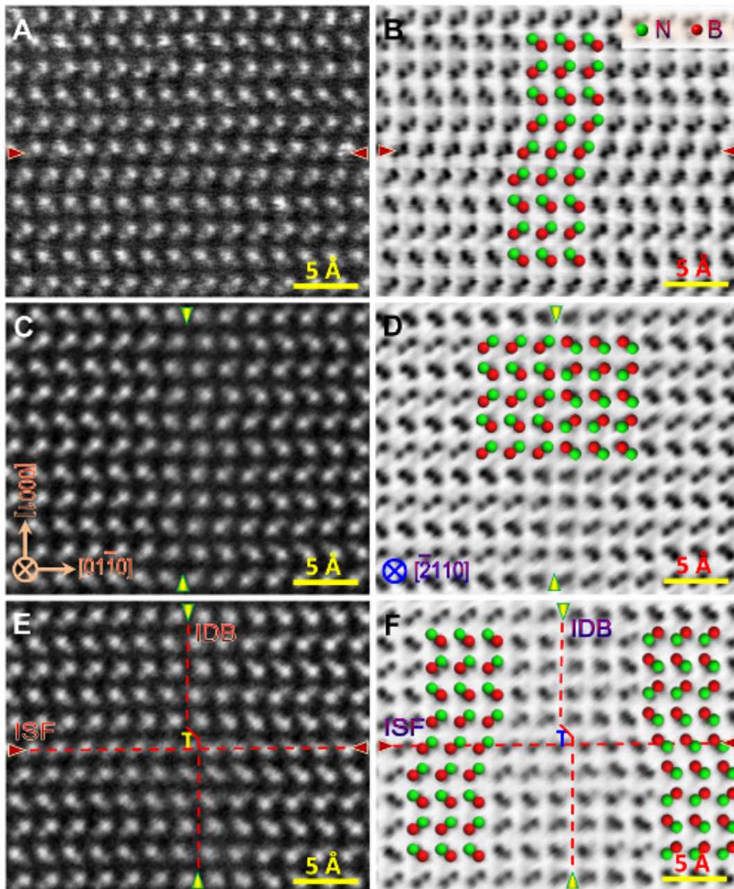
图3、纤锌矿型氮化硼的层错(ISF)和倒反畴界(IDB)的原子结构。(A , B) 层错的HAADF像(A)和相应的ABF像(B)。层错改变了w-BN原子层的堆垛顺序。(C , D) 倒反畴界的HAADF像(C)和相应的ABF像(D)，倒反畴界改变了材料的晶体极性。(E , F) 层错(ISF)和倒反畴界(IDB)交叉区域的HAADF像(E)和相应的ABF像(F)。两组垂直的平面缺陷交叉在一起形成了“层错-倒反畴界结”，并形成了柏氏矢量为 1/3[10-10] 的混合型不全位错。
