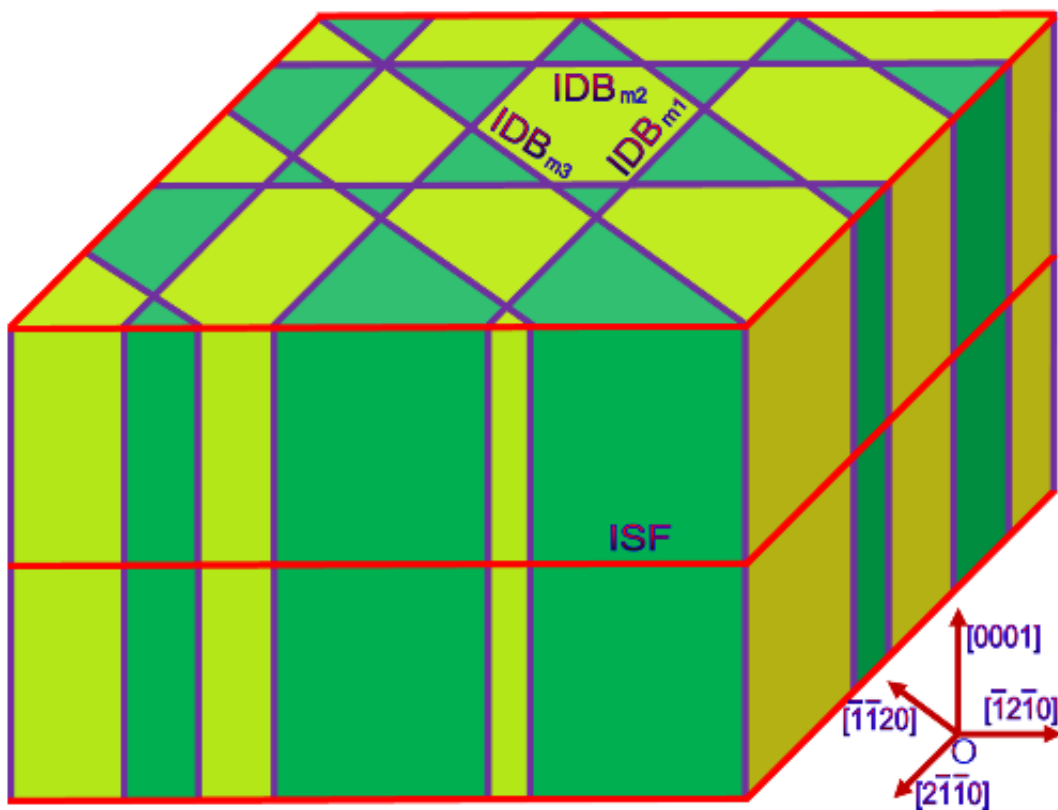
图4、层错(ISF)和倒反畴界(IDB)交织在一起构成三维缺陷网络的示意图。三维缺陷网络将w-BN分割为平均尺寸约十几纳米的棱柱体，相邻的棱柱体具有相反的晶体极性。
