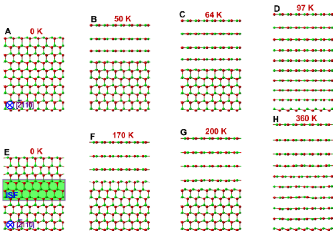
图5、第一性原理分子动力学模拟分析层错(ISF)对w-BN热稳定性的影响。(A – D)完美w-BN的结构演变过程。随着温度的升高，w-BN逐渐转变为类h-BN结构，温度升到97K时相变完成。(E – H
