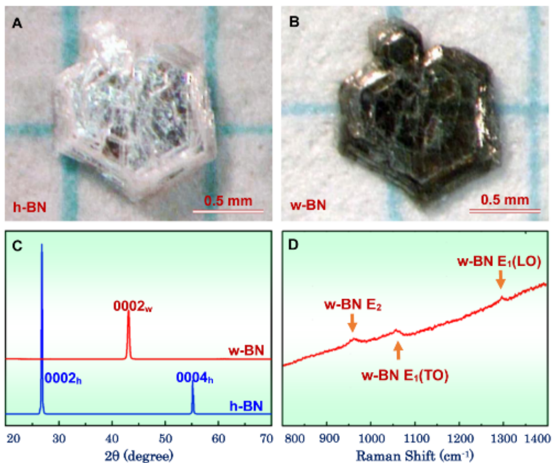
图1、利用六角氮化硼(h-BN)高温高压条件下相变的方法制备的纤锌矿型氮化硼(w-BN)晶体。(A)高质量六角氮化硼单晶，(B)合成的纤锌矿型氮化硼晶体为黑色，(C)晶体相变前后的X射线衍射图；(D)纤锌矿型氮化硼的拉曼光谱。
