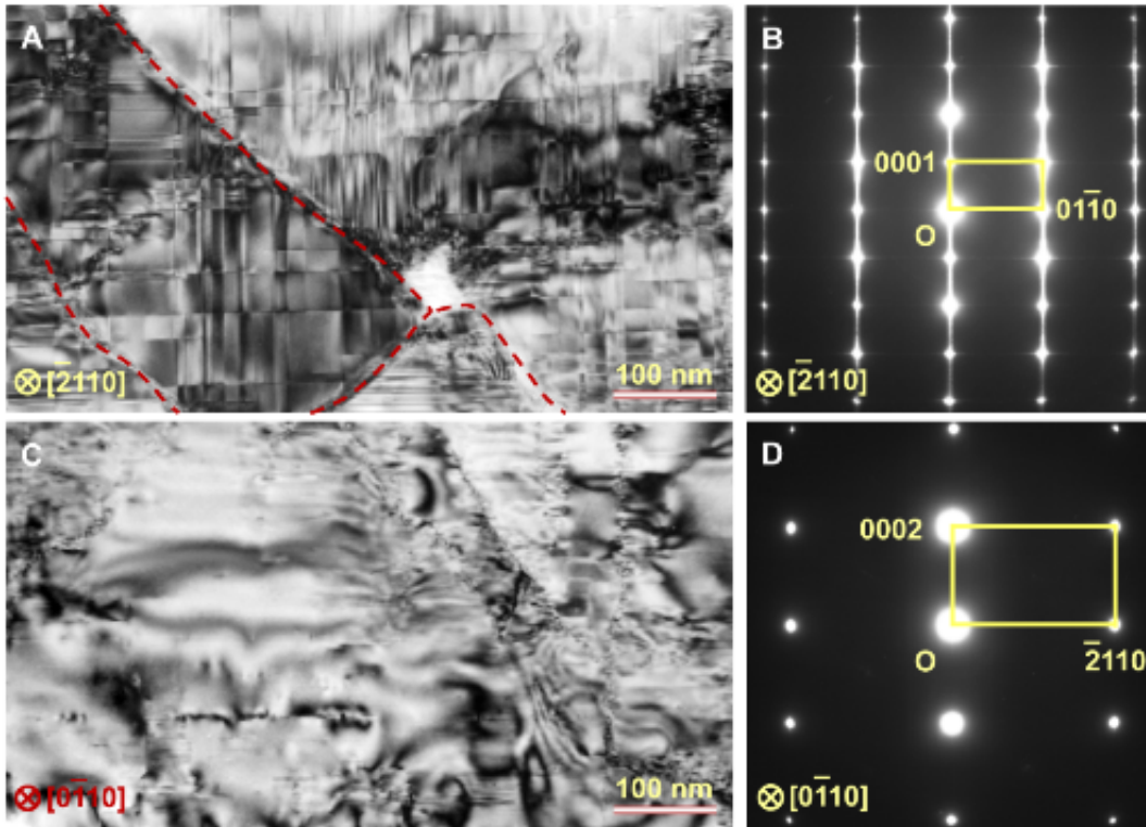
图2、纤锌矿型氮化硼的显微结构。(A , B)沿 [-2110] 晶带轴的TEM明场像(a)和相应的选区电子衍射(b)。材料中形成了(0001)界面上的层错(ISF)和(01-10)棱柱面上的倒反畴界(IDB)组成的两类平面缺陷。红色虚线表示晶界。(C , D)沿 [0-110] 晶带轴的TEM明场像(C)和相应的选区电子衍射(D)。从中可见在 (-2110) 面上没有平面缺陷。
