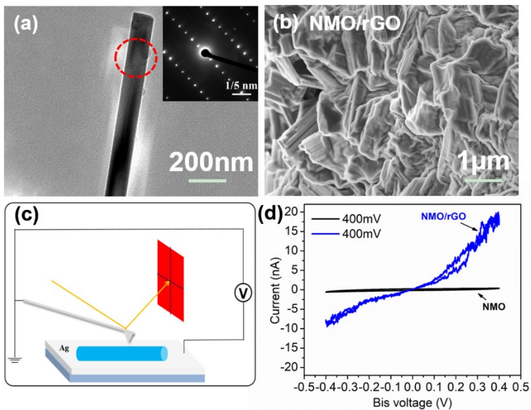
图：Na 0.44 MnO 2 /rGO微观结构及采用c-AFM测量电极材料IV曲线
