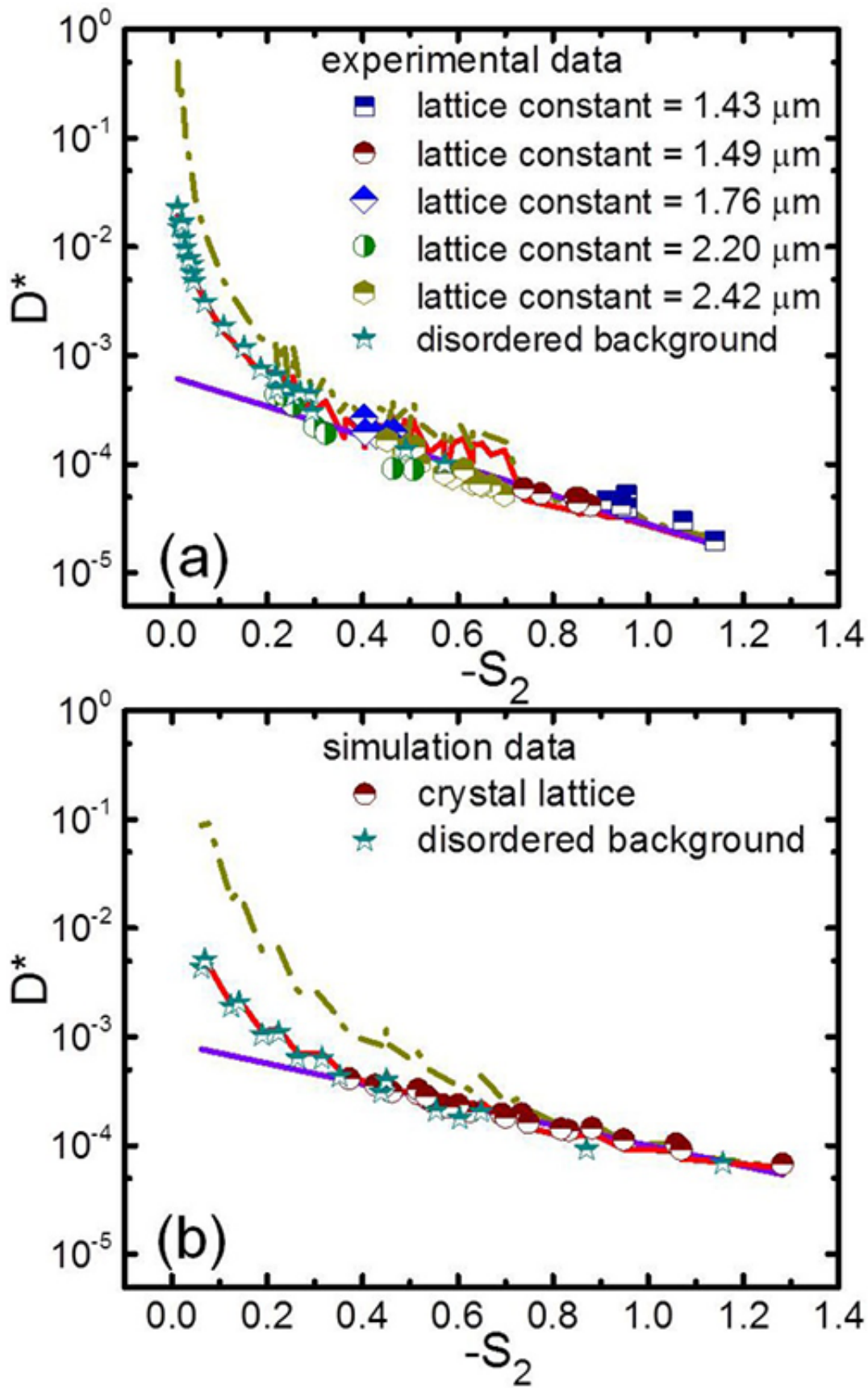
图2. 示踪荧光粒子的无量纲扩散系数 D^* 与两体结构熵 S_2 之间的普适关系。a)实验数据与理论拟合，b)模拟数据与理论拟合。
