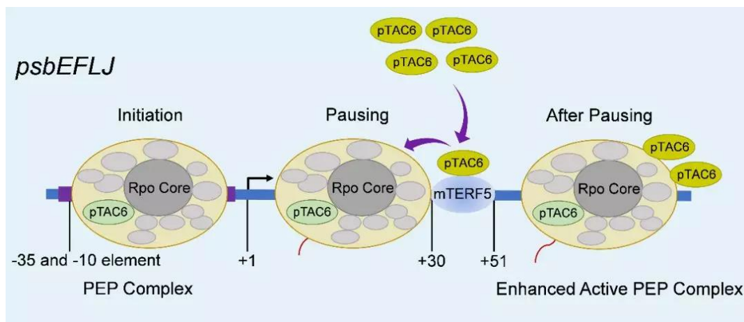
转录暂停因子mTERF5调节叶绿体psbEFLJ操纵子转录的工作模型
